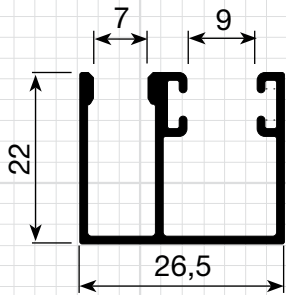
P-203 0,348 Kg/m
