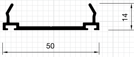
P-878 0,397Kg/m
