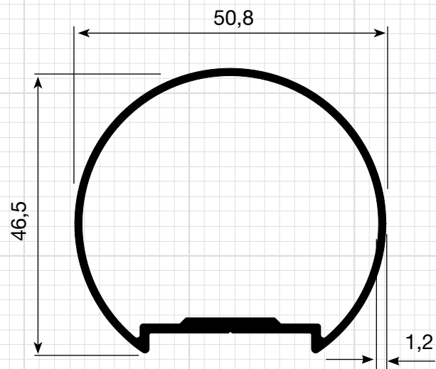
P-333 0,610Kg/m
