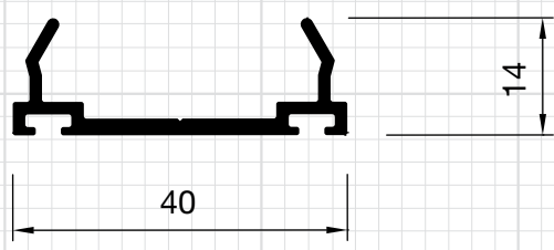
P-35 0,344 Kg/m
