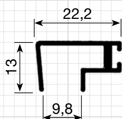
P-266 0,167 Kg/m
