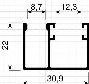
P-207 0,322 Kg/m
