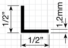
P-226 0,080 Kg/m
