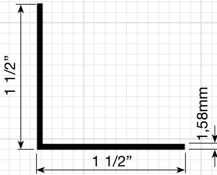
P-296 0,329 Kg/m
