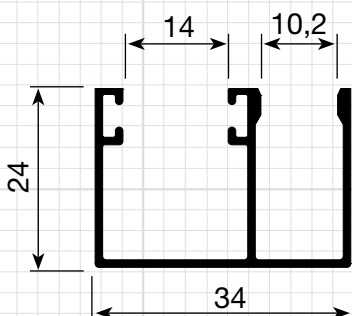
P-05 0,348 Kg/m
