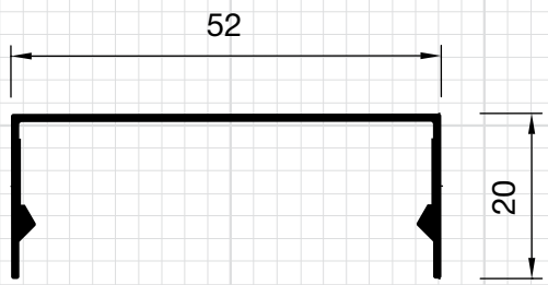
P-877 0,290 Kg/m
