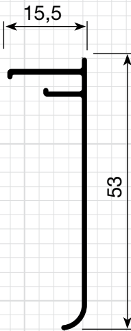
P-360 0,222 Kg/m
