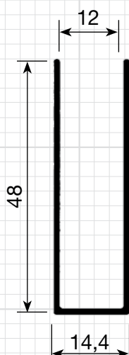
P-254 0,361 Kg/m
