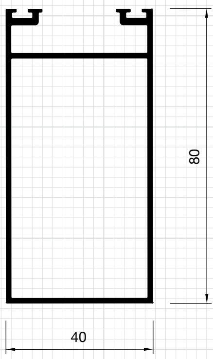
P-36 1,109 Kg/m
