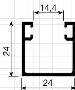
P-06 0,295 Kg/m
