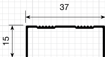
P-372 Perfil de Altura (2x) 0,192 Kg/m
