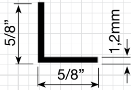
P-227 0,102 Kg/m
