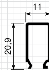
P-260 0,149 Kg/m
