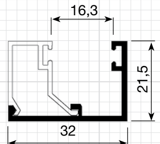
P-26 0,245 Kg/m
