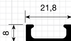
P-371 Perfil Inferior 0,192Kg/m
