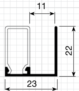
P-259 0,144 Kg/m
