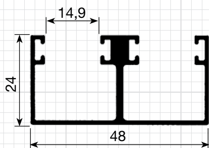
P-253 0,614 Kg/m
