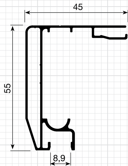
P-205 0,641 Kg/m
