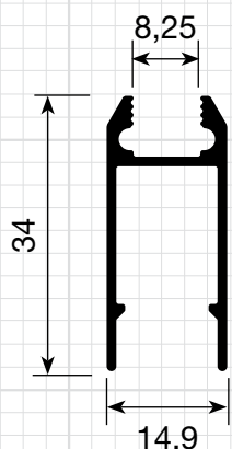
P-370 Perfil Leito 0,319 Kg/m
