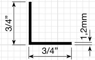
P-330 0,124 Kg/m
