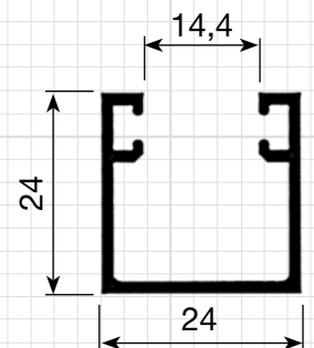
P-06 0,295 Kg/m
