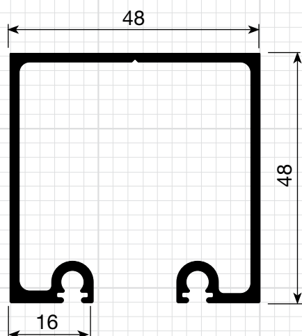
P-373 0,976 Kg/m
