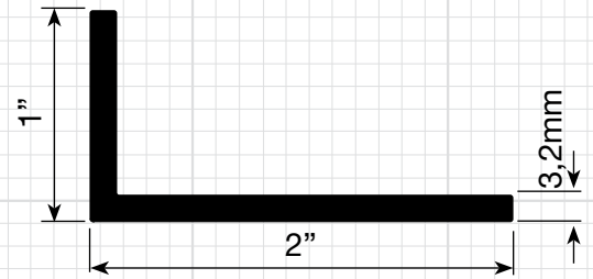
P-353 0,648 Kg/m
