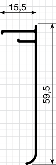
P-364 0,240Kg/m
