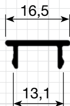
P-211 0,075 Kg/m
