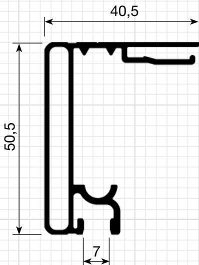
P-307 0,598 Kg/m
