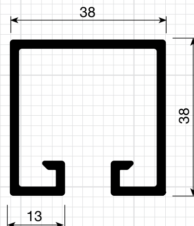
P-37 0,682 Kg/m
