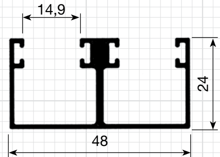
P-253 0,614 Kg/m
