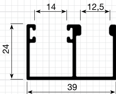
P-210 0,427 Kg/m
