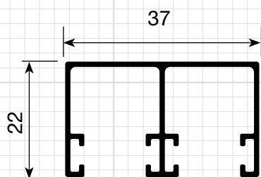
P-369 Perfil Guia Superior 0,371 Kg/m
