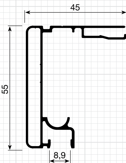
P-308 0,665 Kg/m
