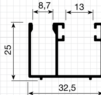
P-323 0,358 Kg/m
