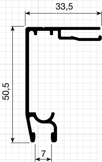
P-201 0,502 Kg/m
