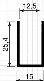
P-10 0,212 Kg/m
